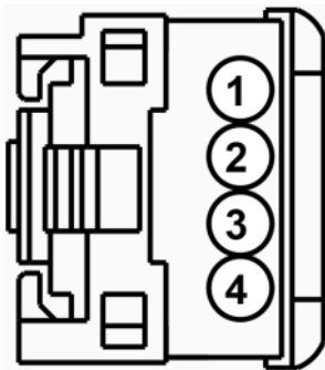
Door Lock Module Connector
