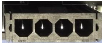
4 Pin Output (J8)
